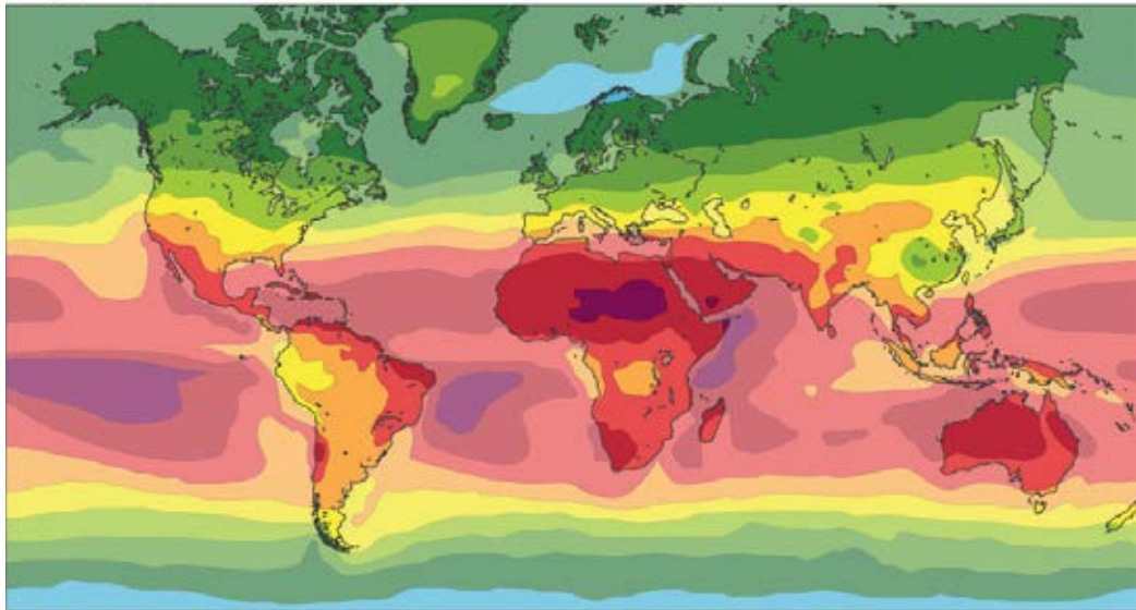
ŞEKİL 1 kLangley Dünya Haritası
